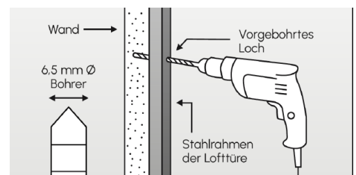
Ściana; wstępnie nawiercony otwór; wiertło Ø 6,5 mm; stalowa rama drzwi.
