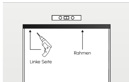
„Linke Seite” - lewa strona; „Rahmen” - rama.
