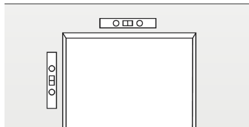
Rysunek: kontrola pionu i poziomu ościeża.
